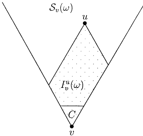
FIG. 4. Region I_v^u(\omega) of \mathcal{S}_v(\omega) .
